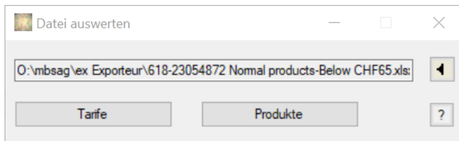
Bild 2 Startfenster
