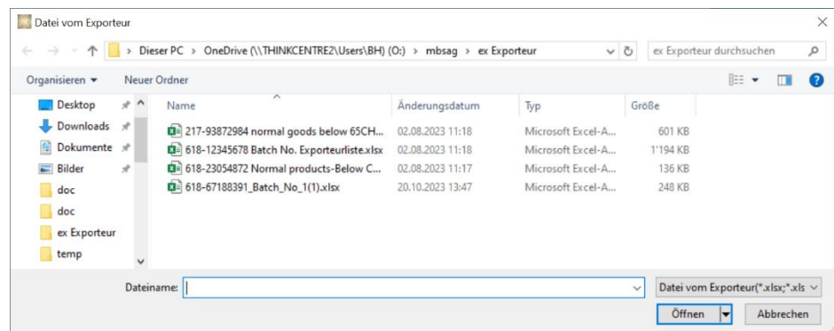
Bild 1 Dateiselektion
